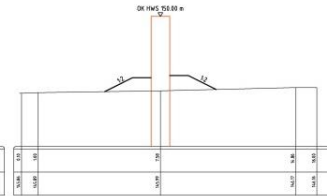
Schnitt E-E
